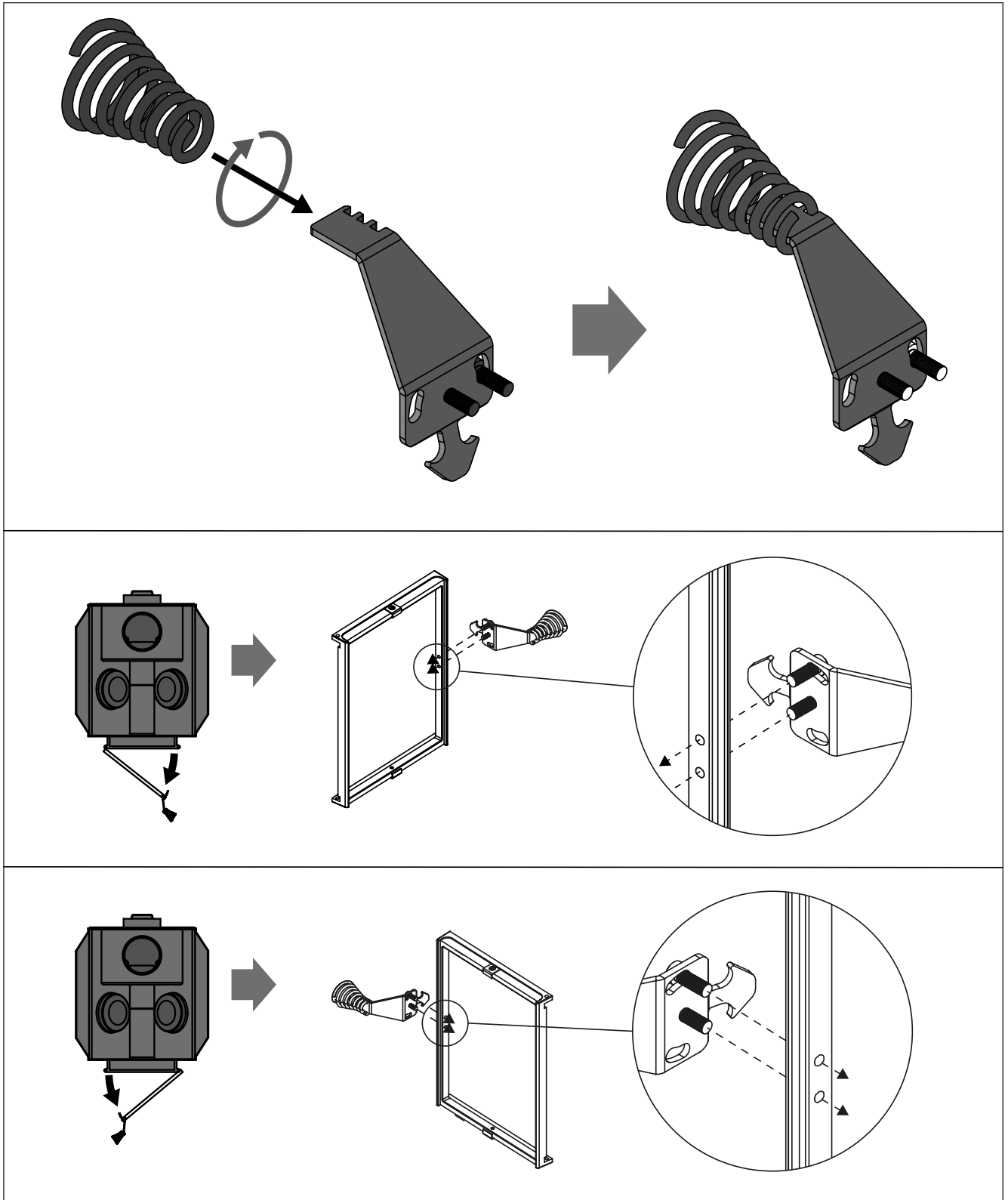
Figure 13. Changing the opening direction of the stove door Abbildung 13. Änderung der Öffnungsrichtung der Ofentür
